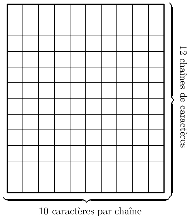
FIGURE 14.1 - Une matrice de caractères
